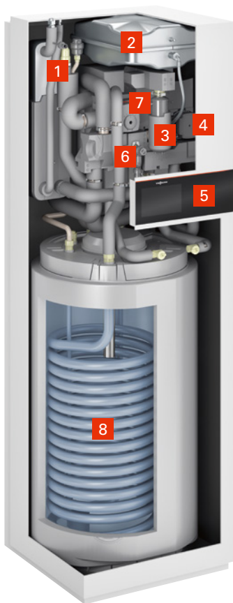
VITOCAL 222-S Med en värme-/kylkrets
