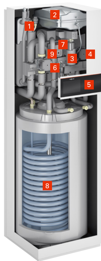
VITOCAL 222-S Med två värme-/kylkretsar
