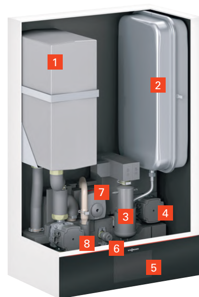
VITOCAL 250-A Med två integrerade värme-/kylkretsar
