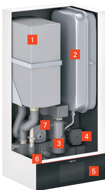
VITOCAL 250-A Med en integrerad värme-/kylkrets
